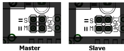
Рис. 8: Конфигурация UART
