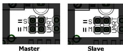
Рис. 8: Конфигурация UART
